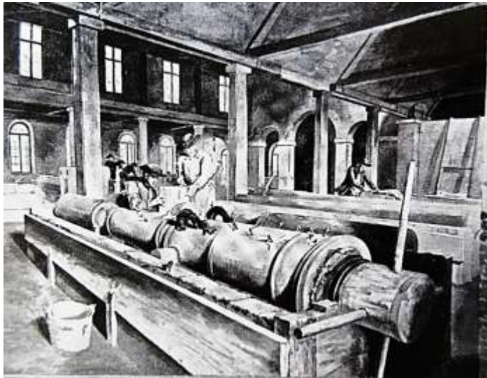
Het vormen van geschut aan de horizontale spil in de gieterij te Woolwich. Naar een tekening van Pieter Verbruggen uit ca. 1775. →
